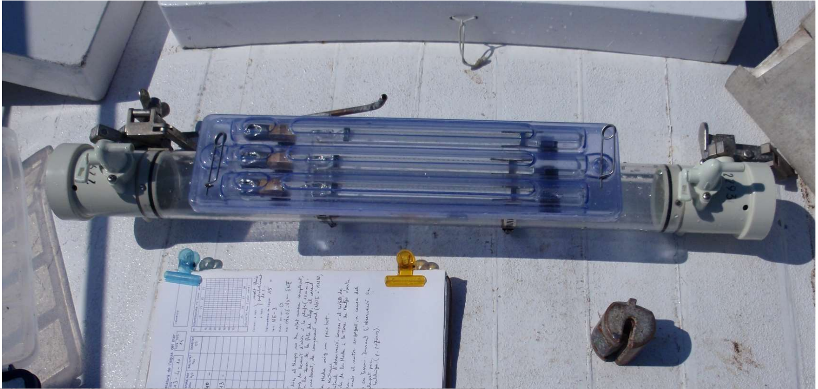
Aparells per a la mesura de la temperatura de l'aigua del mar
