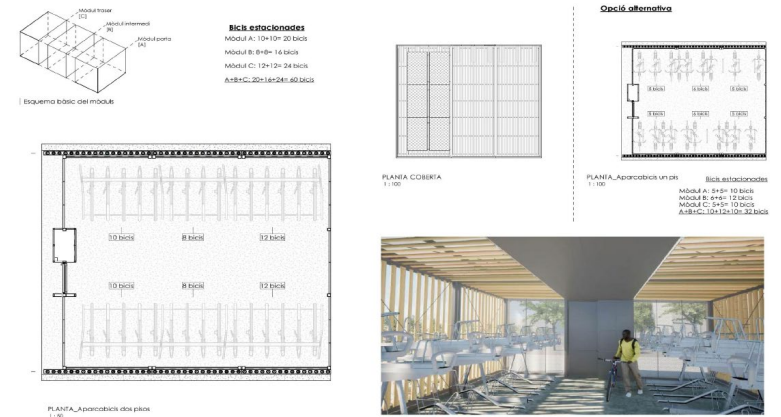
2.12 Planta BICITANCAT 6x6 sólo aparca bicicletas
