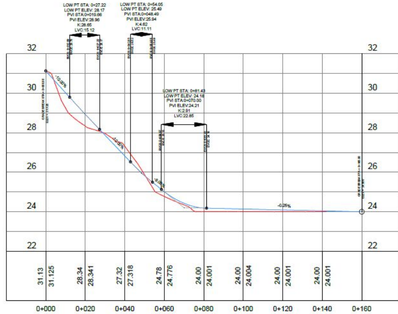
SECCIÓ LONGITUDINAL
